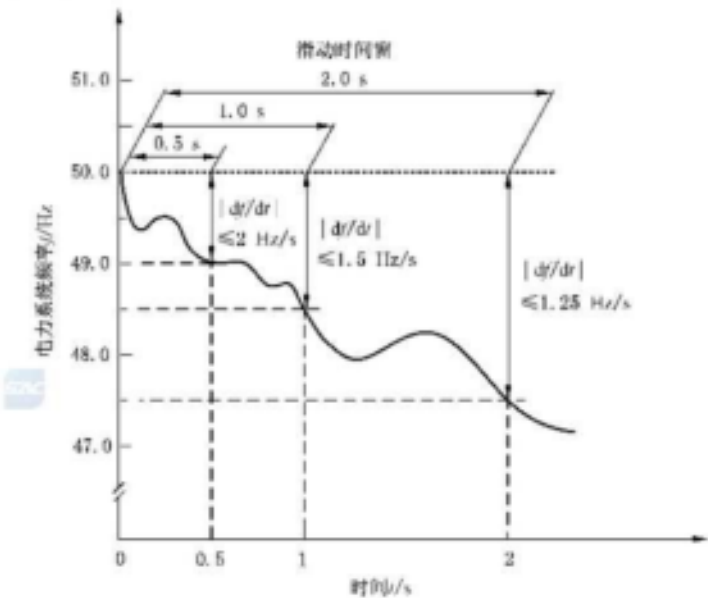
图 4 滑动时间窗与频率变化率示意图
